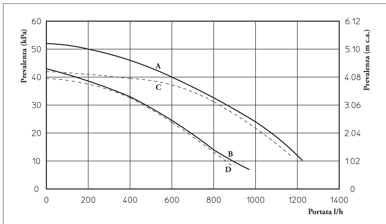
GRUNDFOS UPS 15-50 AO
